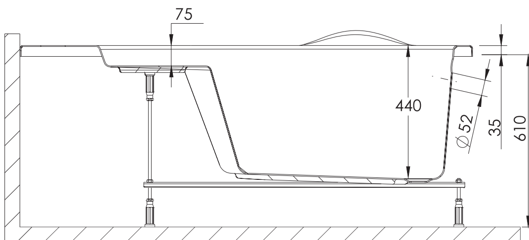
ŘEZ A-A
